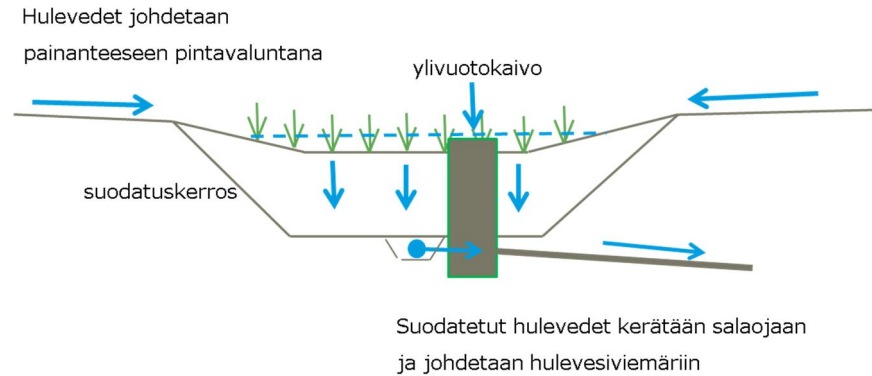
Kuva 19. Hulevesien viivytytys- ja suodatuspainanne, joka soveltuu myös huonosti vettä johtavalle maalle
